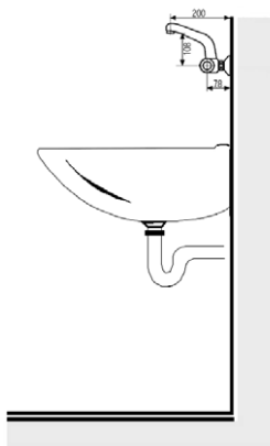
Abmessungen 207 für zentrale Warmwasserversorgung
